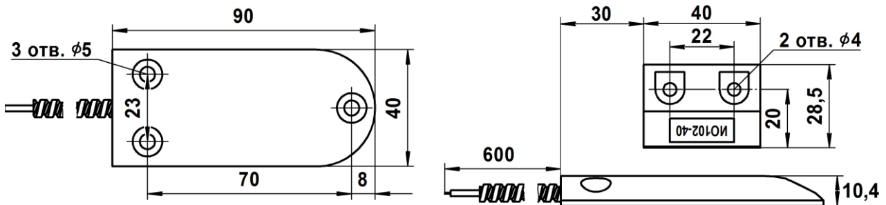
Рисунок 1 – Извещатели модификаций А2П, А2М, А3П, А3М
